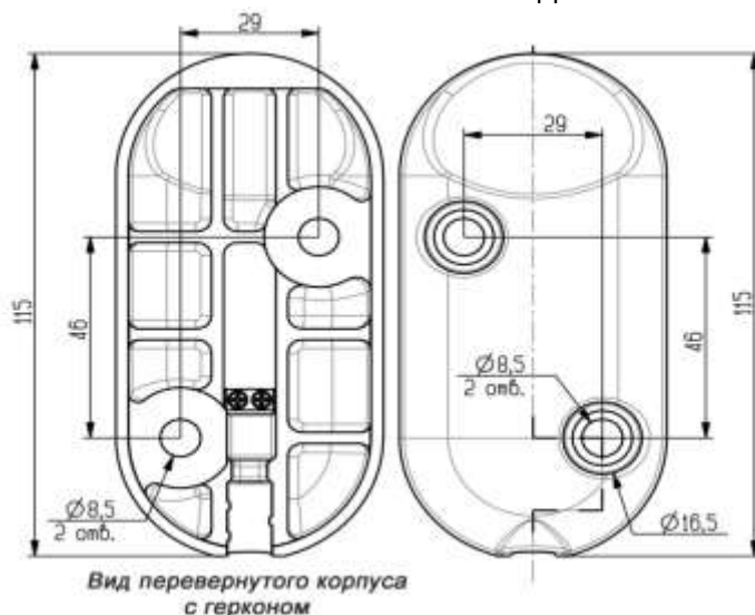
рис.1. Габаритные и установочные размеры. Высота задающего и исполнительного блока – 14 мм.
