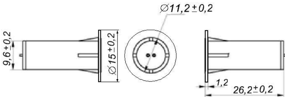
рис.1. Габаритные и установочные размеры
