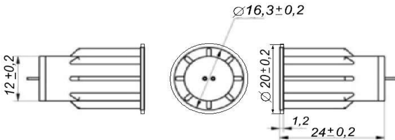
рис.1. Габаритные и установочные размеры
