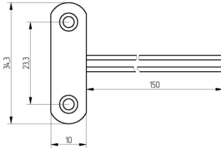
Рис. 1. Габаритные и установочные размеры.
