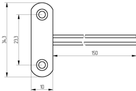
Рис. 1. Габаритные и установочные размеры.
