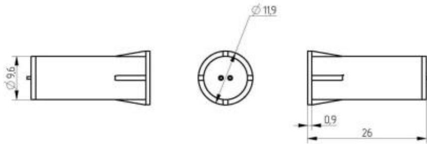
Рис.1 Габаритные и установочные размеры.
