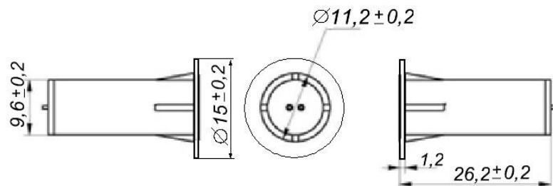
Рис.1 Габаритные и установочные размеры.
