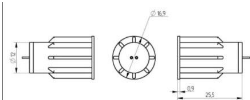
Рис. 1 Габаритные и установочные размеры.
